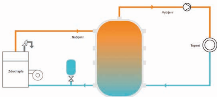
Základní princip funkce akumulaci nádob. Zdroj: Akumulační zásobníky. Výměníky tepla. ( http://www.reflexcz.cz )
